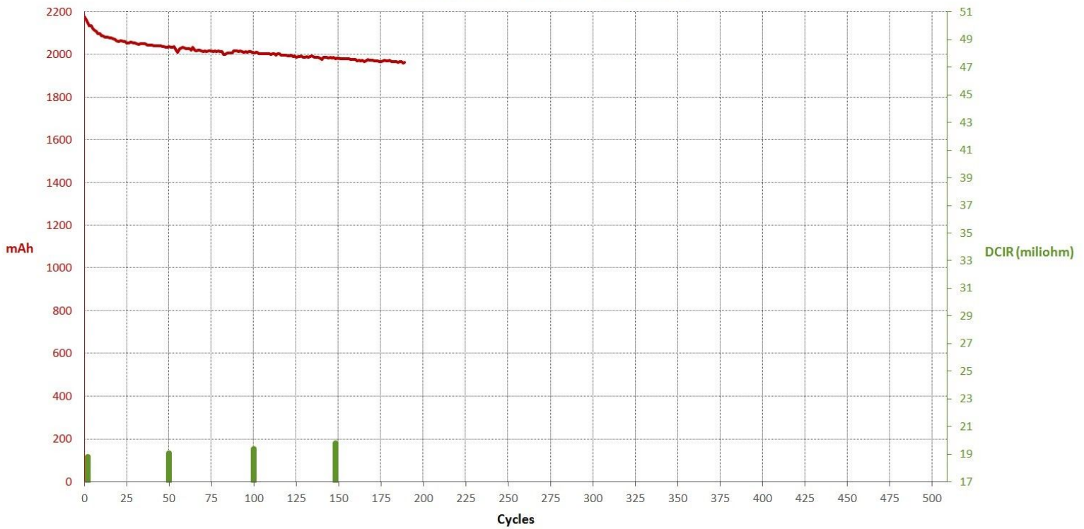
Samsung 30Q No3 cycling 4,1 - 3,3 V 2,5/1 A
